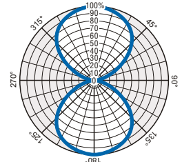
CHARAKTERYSTYKA KIERUNKOWA VHF
